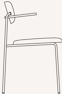
P6-006 W57/D52/H80 SH48
