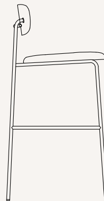
P6-012 W45/D52/H102 SH77
